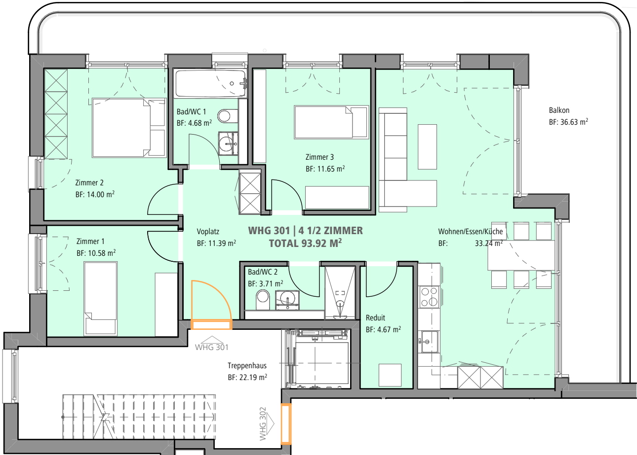
Grundriss 3.OG
